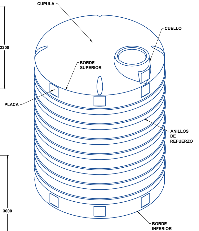
VISTA ISOMETRICA
