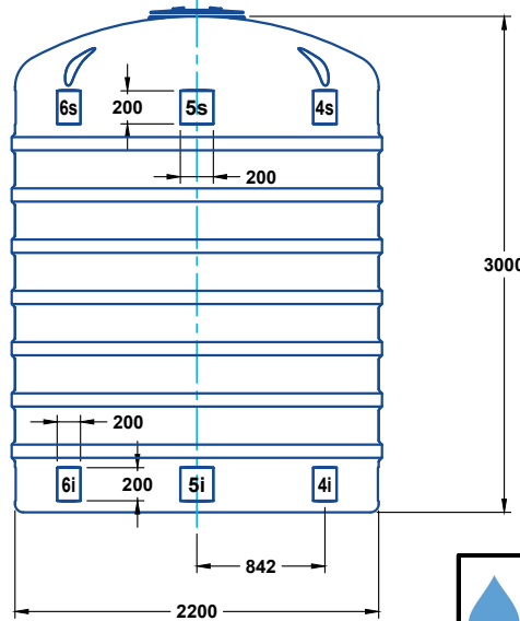
VISTA POSTERIOR
