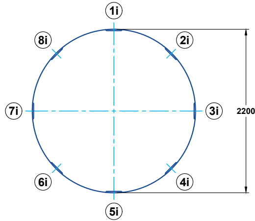
VISTA INFERIOR
